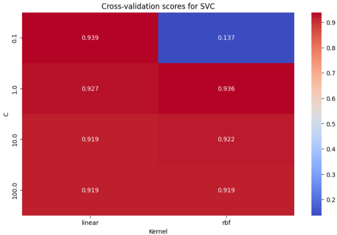
Hình 3.4 Quá trình đánh giá để chọn ra siêu tham số
