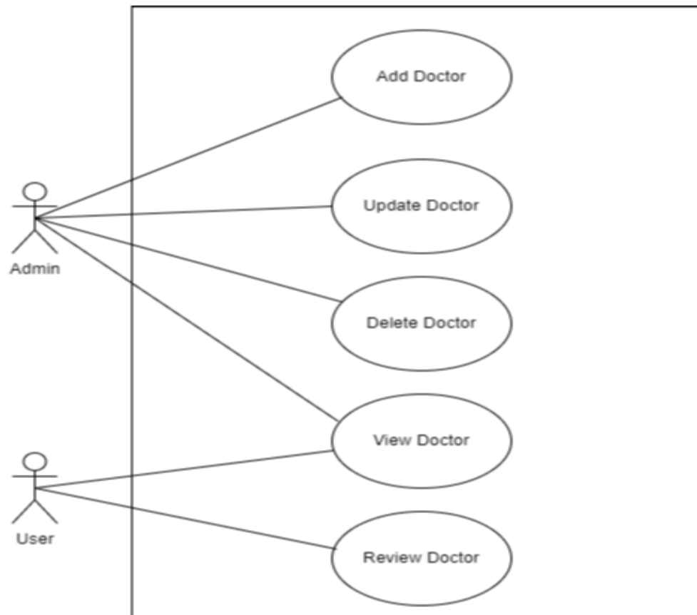
Hình 2.3 Sơ đồ usecase về bác sĩ
