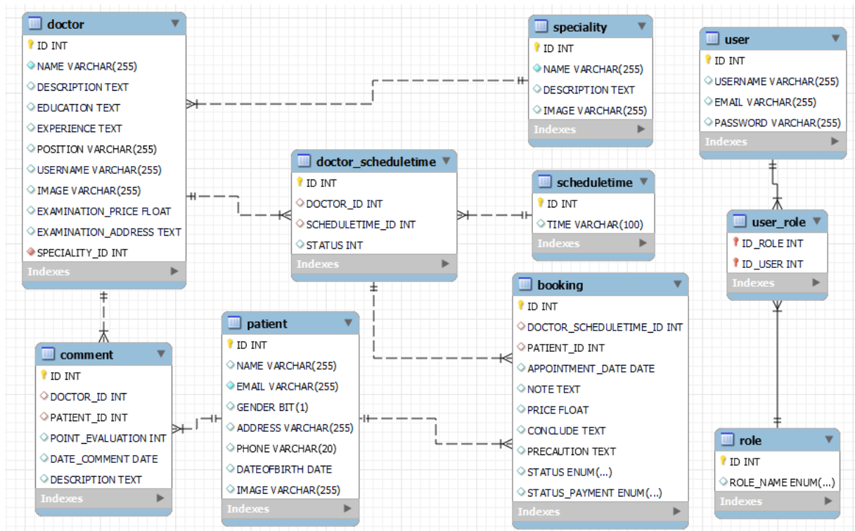
Hình 2.7 Cơ sở dữ liệu của hệ thống
